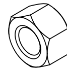
4X. HEX NUT (1/2"-13 TPI. )
