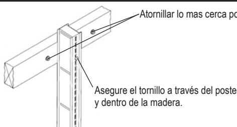
TROZO DE MADERA DE 5cm x 10cm CONTINUA DETRAS DEL POSTE
