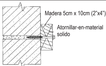
LADRILLOS (Block de concreto, ladrillo etc)
