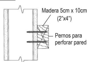
PARED CON MARCO DE METAL
