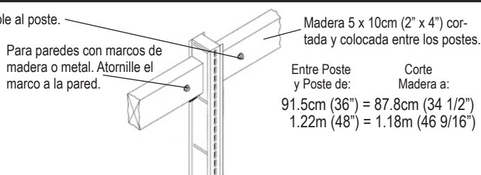
TROZO DE MADERA DE 5cm x 10cm ENTRE POSTES
