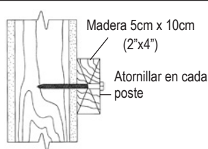
PARED MONTANTE DE MADERA
